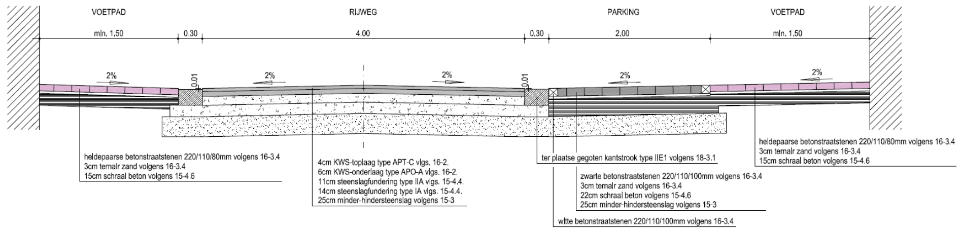
MODEL DWARSPROFIEL TYPE 1:
